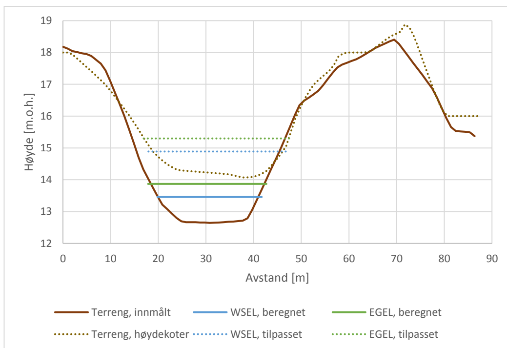
Figur 9: Tverrprofil 401.
